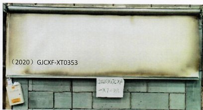
照片2 耐高温性能试验后试件情况
